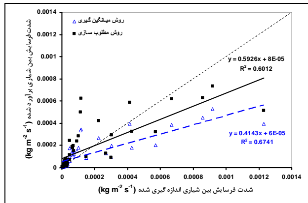
شکل 4- مقادیر اندازه‌گیری شده و برآوردی فرسایش بین شیاری با استفاده از مدل WEPP پس از واسنجی به دو روش میانگین‌گیری و مطلوب‌سازی در تمامی تنش برشی‌ها
