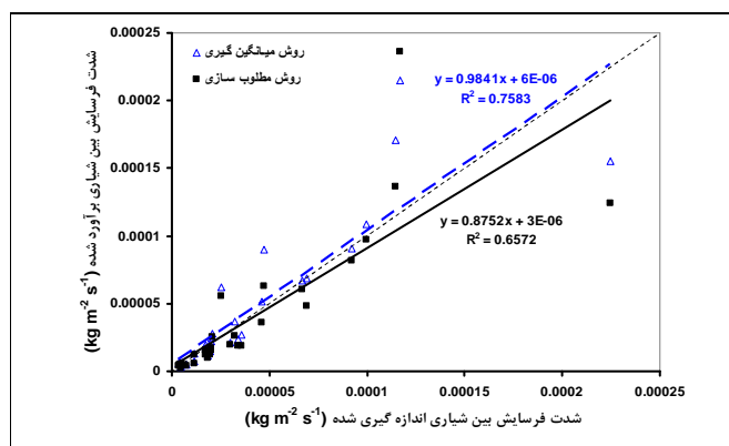
شکل 3- مقادیر اندازه‌گیری شده و برآوردی فرسایش بین‌شیاری با استفاده از مدل WEPP پس از واسنجی به دو روش میانگین‌گیری و مطلوب‌سازی در تنش برشی‌های کمتر از آستانه
