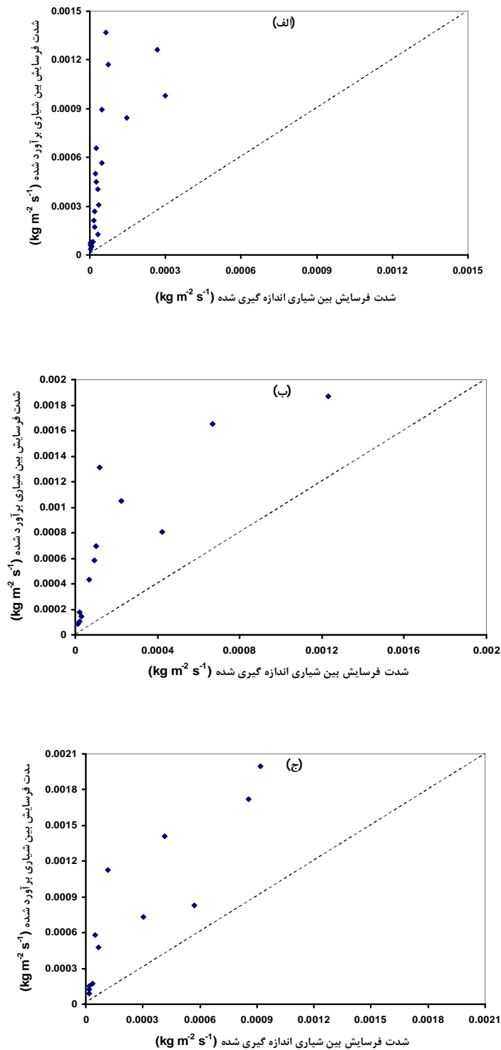
شکل 2- مقادیر اندازه‌گیری شده و برآوردی شدت فرسایش بین‌شیاری با استفاده از مدل WEPP قبل از واسنجی، در تمامی تنش برشی‌ها برای؛ (الف) خاک هشتگرد، (ب) خاک دانشکده و (ج) خاک سهیلیه
