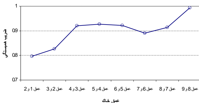
شکل 7- تغییرات ضریب همبستگی بین شوری عصاره اشباع خاک در هر دو عمق مجاور یکدیگر در دشت آزادگان - استان خوزستان. عمق 1 مربوط به خاک لایه سطحی (0-30 سانتیمتر) و عمق 9 مربوط به لایه عمیق خاک (270-240 سانتیمتر) می باشد.
