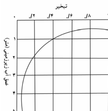
شکل ۵- رابطه شماتیک بین عمق آب زیر زمینی و نرخ نسبی تبخیر از سطح خاک
